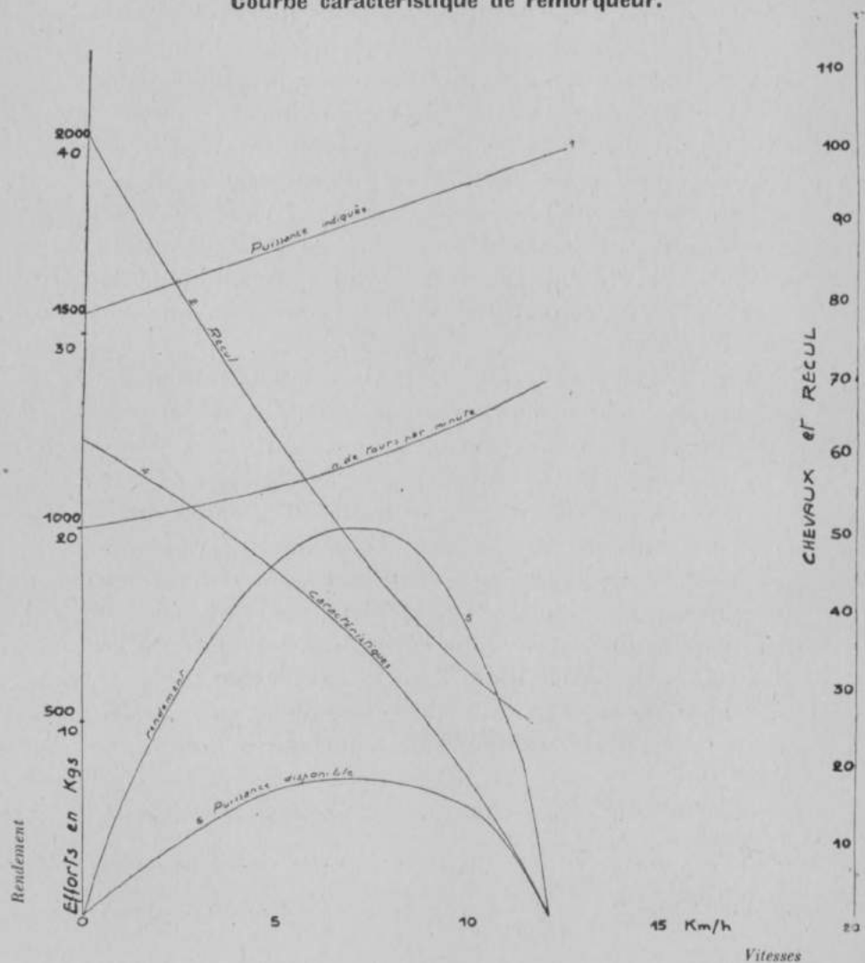
Courbe caractéristique de remorqueur.
