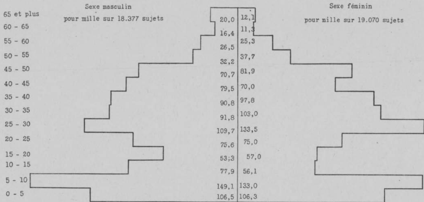
Pyramide des âges par sexes et par groupes de 5 en 5 ans.
