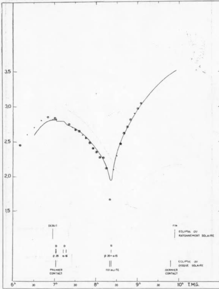
FIG 7. — Bangui, 25 février 1952, fréquences critiques de la couche E.
