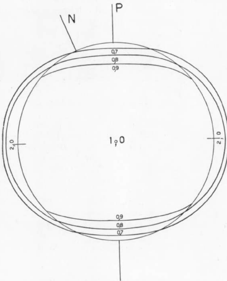
FIG. 2. — Modèle solaire.
