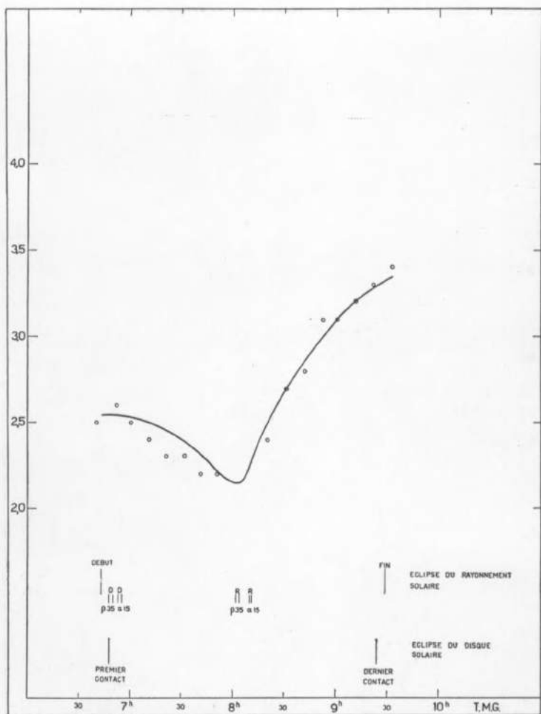
FIG. 8. — Léopoldville, 25 février 1952, fréquences critiques de la couche E.
