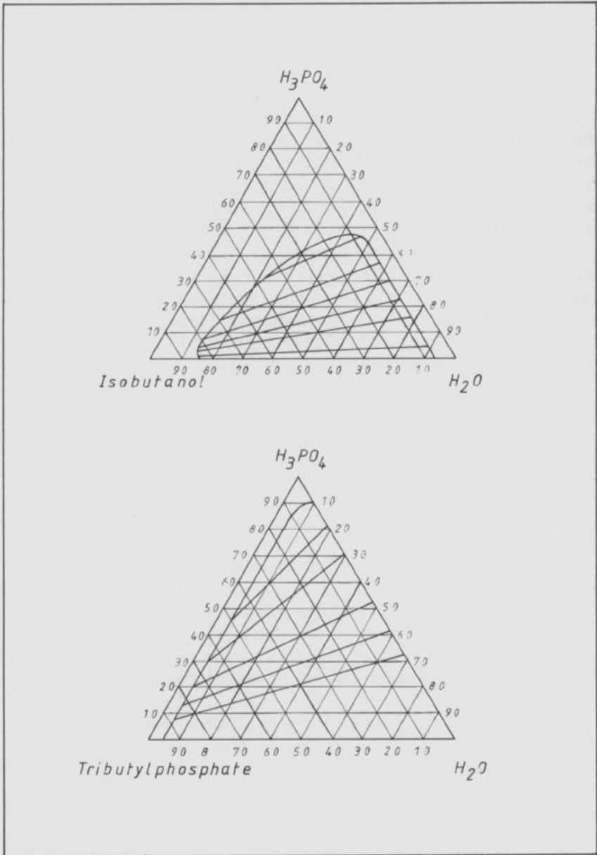
Fig. 2. Diagrammes d'équilibre du système ( H_3PO_4 - H_2O - Solvant) pour l'isobutanol et le tributylphosphate à 25^\circ C .
