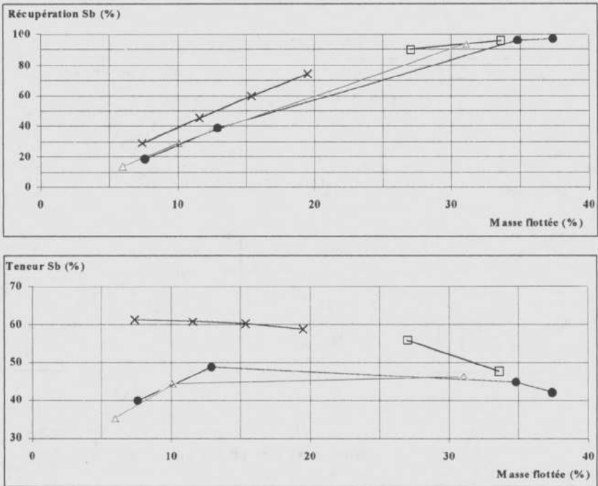
Fig. 8. — Résultats des essais de flottation (partie ébauchage).
