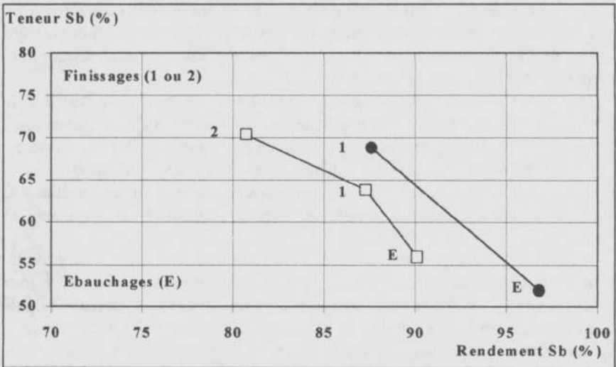
Fig. 9. — Résultats des essais de finissage.
